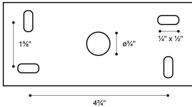
Anchor Bolt Template.
